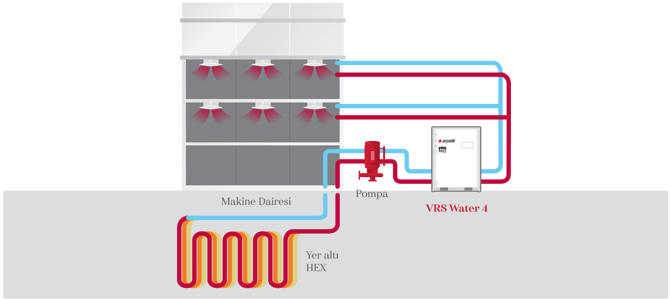
Soğutucu - FCU
